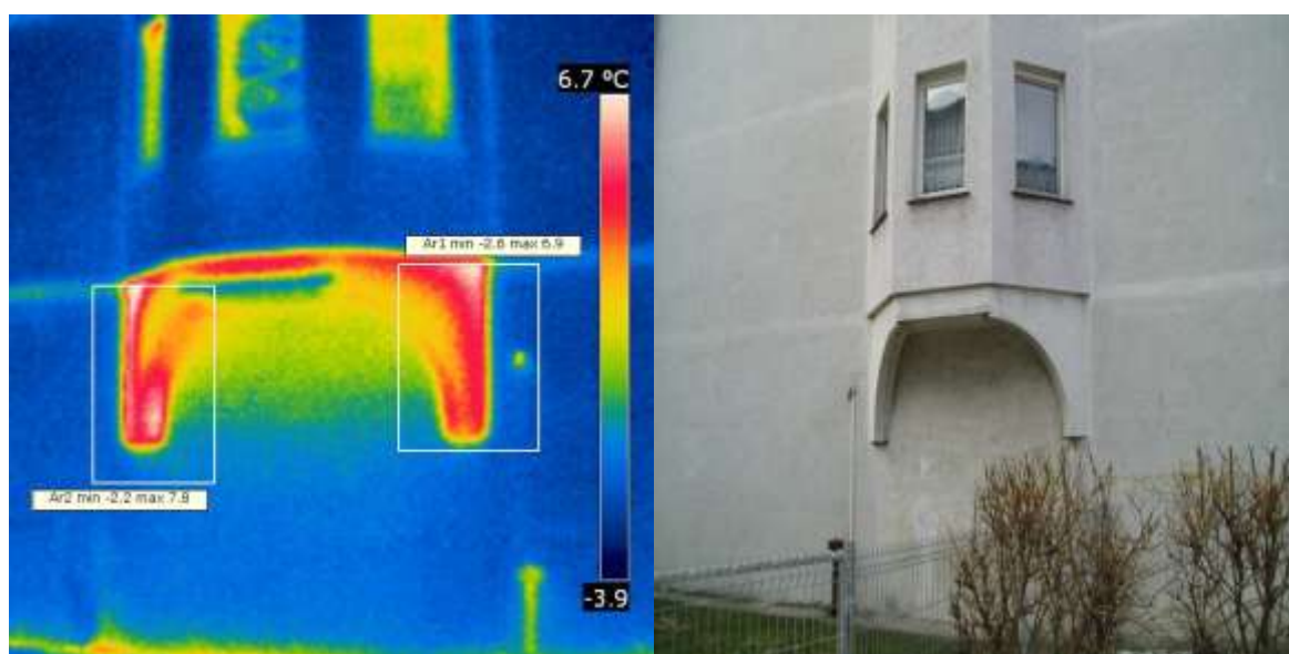
Rys. 19 Termogram nieizolowanej podpory żelbetowej wykusza
